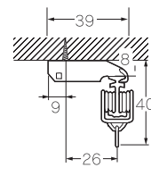
天井シングルワンタッチブラケット付
