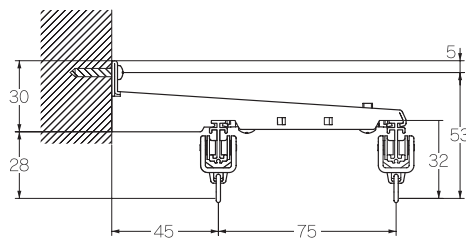
LWワンタッチブラケット
