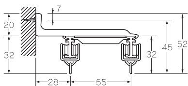
正面ダブル付
