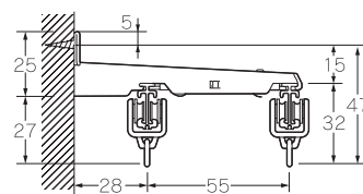
正面ダブルワンタッチブラケット付
