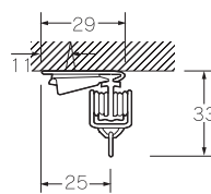
天井シングル付
