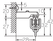
正面シングルワンタッチブラケット付
