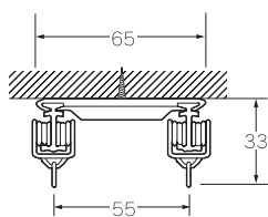
天井ダブル付
