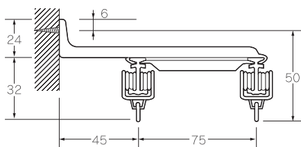
正面LWブラケット付(公団仕様A2型)
