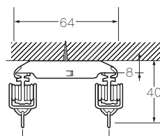
天井ダブルワンタッチブラケット付
